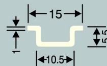
DNR - 15 Mini Rail 5.5 x 15 x 1 mm
